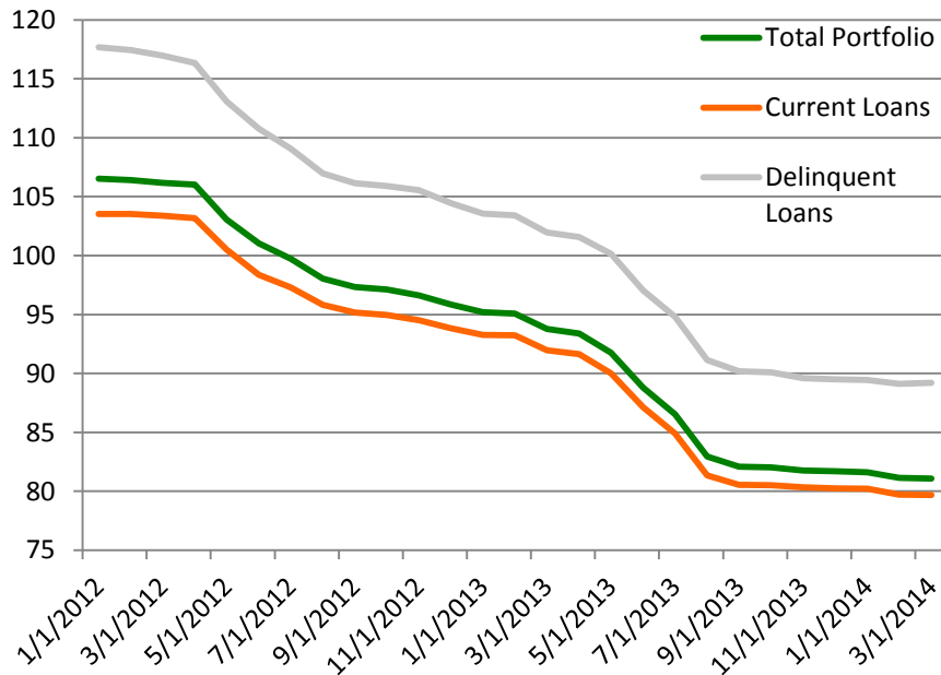
LTV Trend
